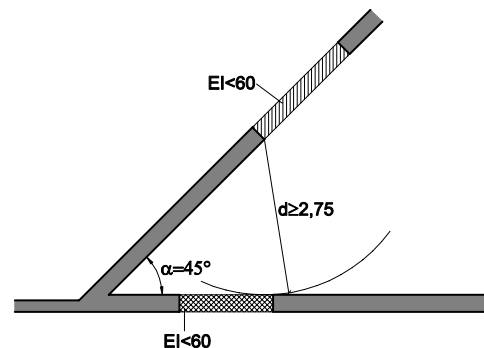
Figura 1.2. Fachadas a 45°
