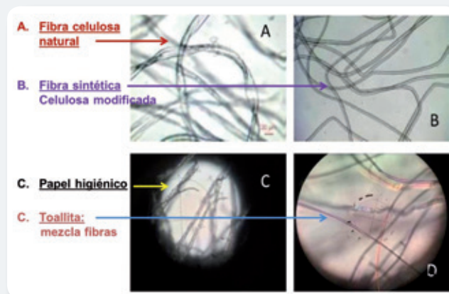
Figura 2: Investigación microscópica de las fibras de toallitas y papel higiénico. Figure 2: Microscopic study of wipe and toilet paper fibres.
