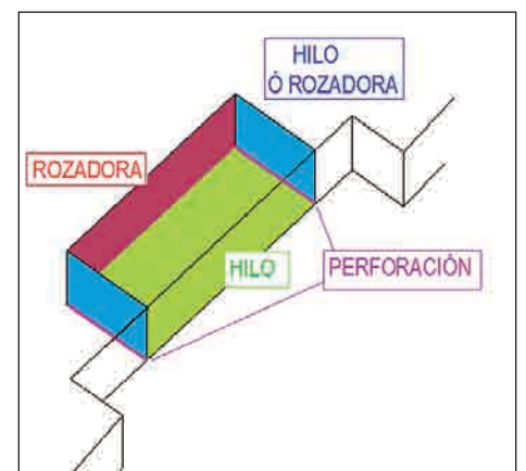
■ [Fig. 8] .- Levantes mediante corte para independizar una masa estéril de capa a volar.
