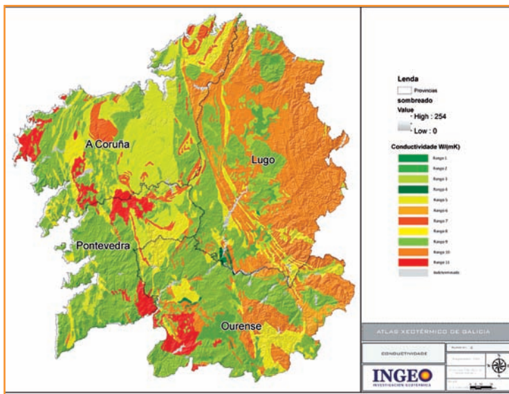
■ [Figura 1] .- Mapa de conductividad térmica del subsuelo gallego.
