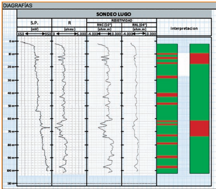
■ [Figura 4] .- Diagrama de resistividad geofísica.
