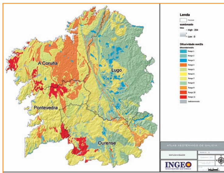
■ [Figura 2].- Mapa de difusividad térmica del subsuelo gallego.
